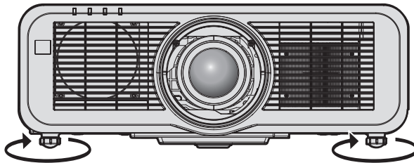
Максимальный диапазон настройки Регулируемые ножки: 23 mm (29/32") каждая
