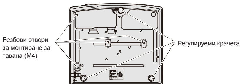
Позиции на резбовите отвори за монтиране за тавана и регулируемите крачета
